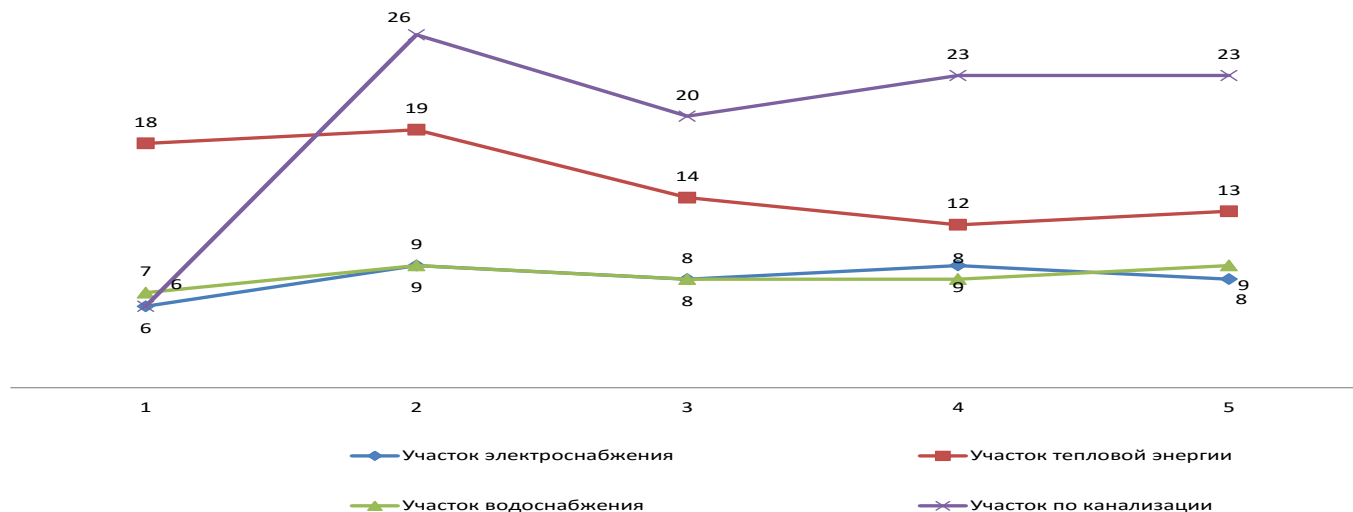
Анализ аварийности сетей по ЦТВЭС за период с 2014-2018гг.
